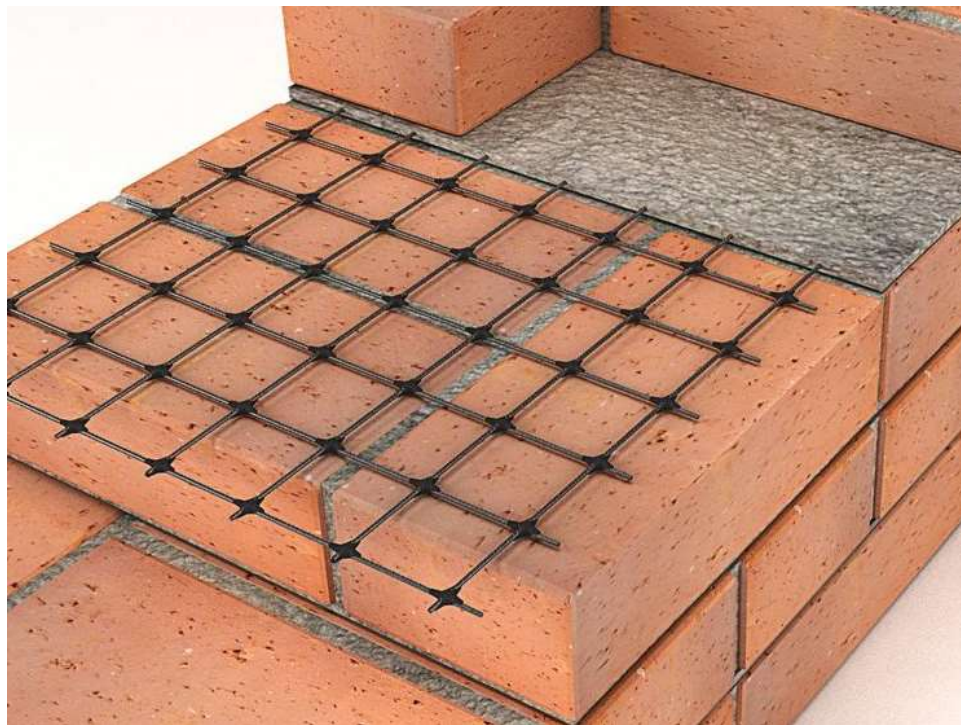
Армирование кирпичных кладок композитными сетками
